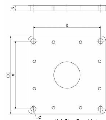
Nr4 Chevilles chimiques
