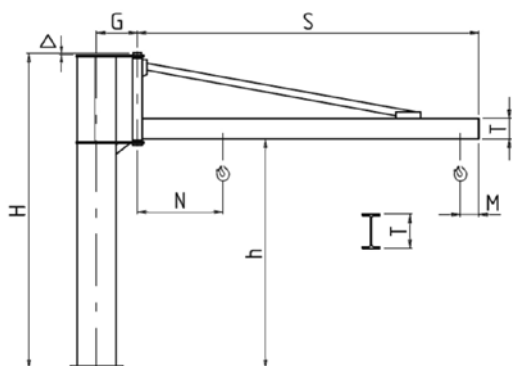
300° Potence sur fut - Rotation 300°
